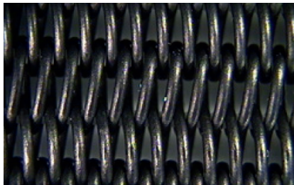
Abb. 5: Spiralsieb aus 100 % AntiStat
