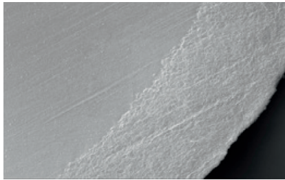
Abb. 2: Übergangsbereich Kern/Mantel
