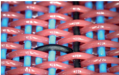
Abb. 4: Siebgewebe aus PET mit AntiStat in Kett- und Schussrichtung
